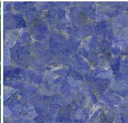
Lapis Lazuli
