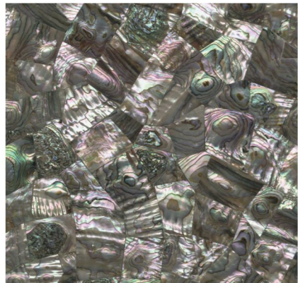
Abalone
